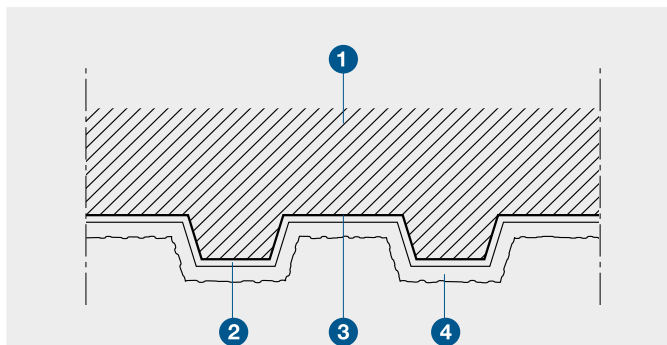
Detalle sección transversal
