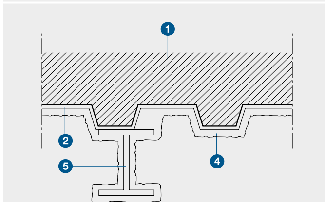
Detalles de protección conjunta forjado/estructura metálica
